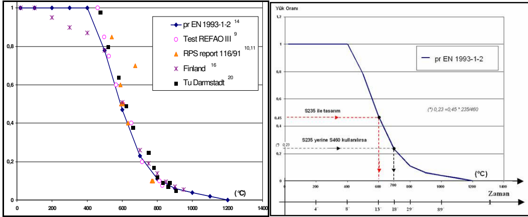
Şekil 5 Sıcaklığın fonksiyonu olarak etkin akma dayanım azalımı.
