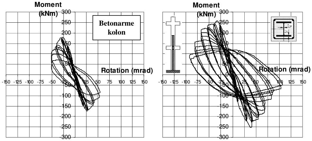
Şekil 12 Çiine çelik profil yerleştirilen betonaarme kolonun moment-dönme grafiği.
