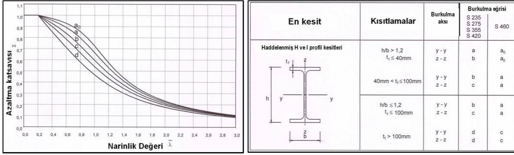
Şekil 4 Eurocode'a göre burkulma eğrileri.
