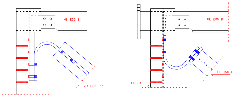
Şekil 11 U form birleşim ile iki farklı tasarım.
