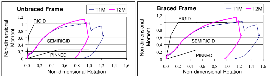
Şekil 14 Eurocode 3'e göre birleşim sınıflandırması.
