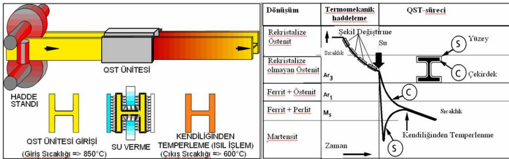
Şekil 1 QST sürecinin ve ısı akışının şematik gösterimi.
